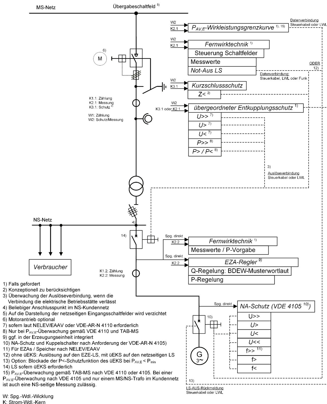
Bild D.22 Mischanlage – Beispiel für eine an das Mittelspannungsnetz angeschlossene Kundenanlage mit Bezug und Erzeugungsanlage, Lasttrennschalter und einer Erzeugungsanlage mit Zertifizierung nach VDE-AR-N 4105 [3] oder Anschluss nach NELEV/EAAV-2024 (Bild 1.1 der Ergänzungen [2]) (ohne Inselbetriebsmöglichkeit, Anschluss nicht in UW bzw. Schaltstation) vorbehaltlich anders lautender Hinweise des VDE/FNN
