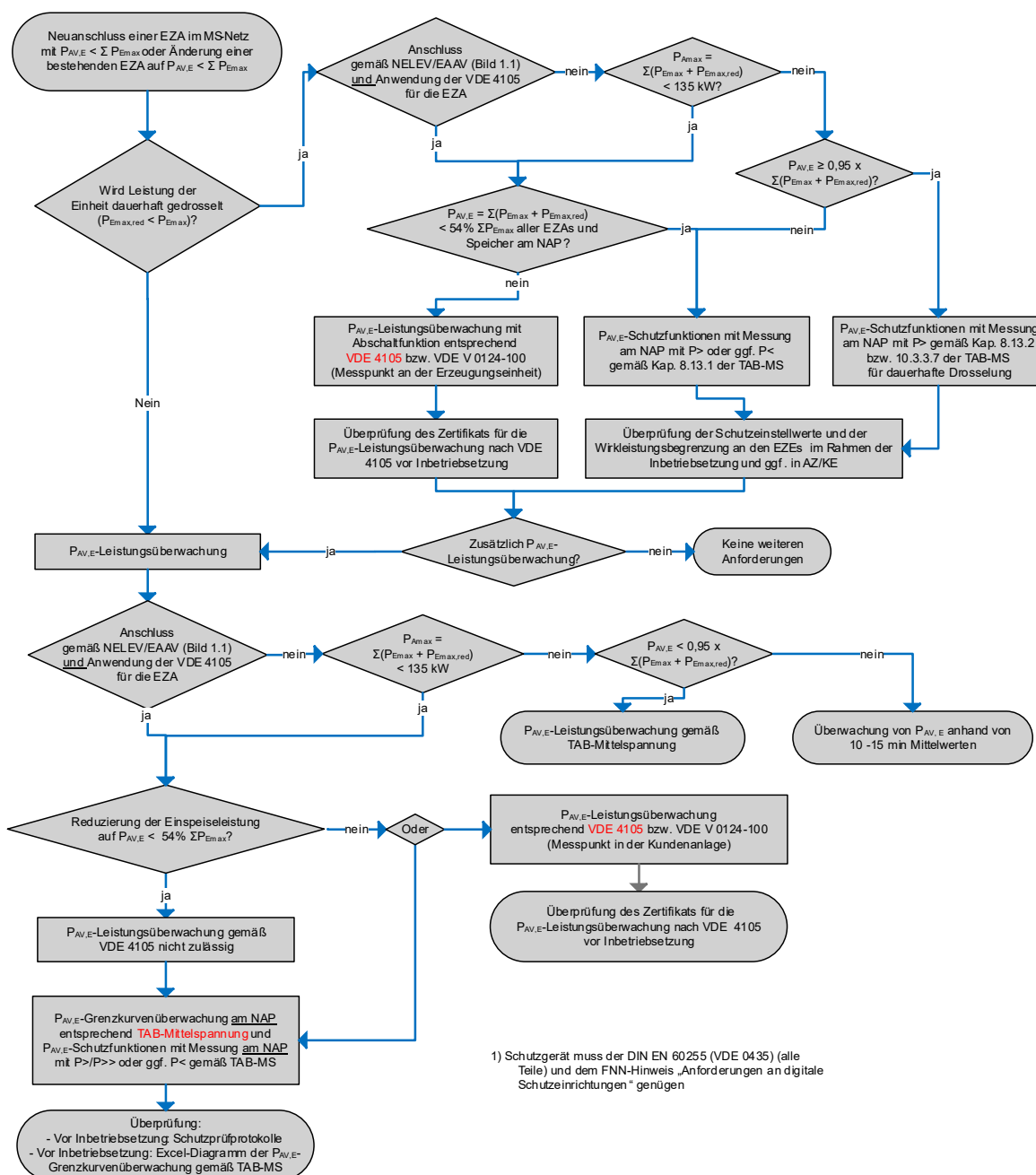
Bild 8.1 Prinzipielle Übersicht der Anforderungen an Erzeugungsanlagen / Speicher mit P_{AV,E} < \Sigma(P_{E\max} + P_{E\max,red}) am Netzanschlusspunkt und/oder bei Erzeugungseinheiten mit einer dauerhaften Drosselung P_{E\max,red} < P_{E\max}
