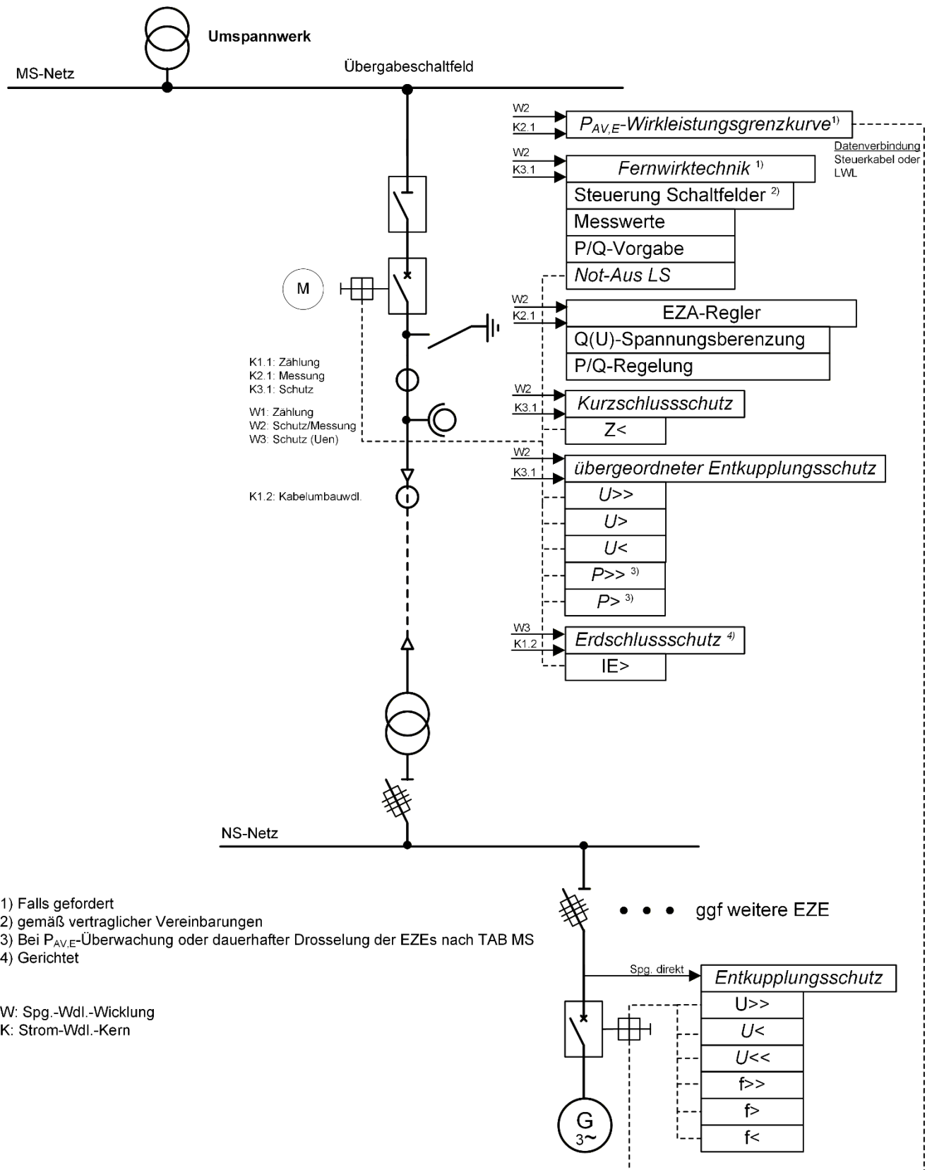
Bild D.15 Einspeisung – Beispiel einer an ein Umspannwerk mittelspannungsseitig angeschlossenen Erzeugungsanlagen im UW-Schaltfeld mit Leistungsschalter und Erzeugungseinheit ohne Inselbetriebsmöglichkeit
